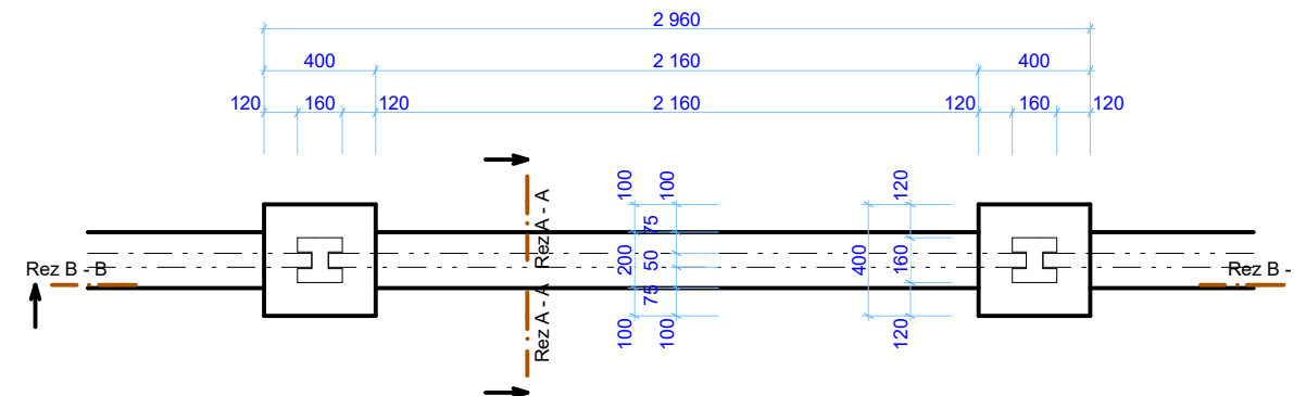
PÔDORYS ZÁKLADOV
